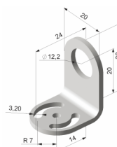
固定安装支架
