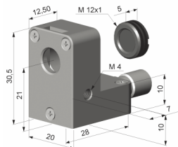
空气吹扫器
